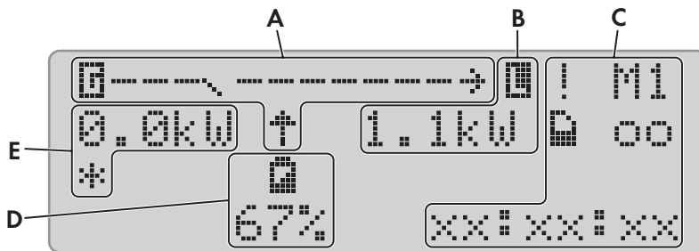
Abbildung 6: Energieflüsse und Status des Wechselrichters Sunny Island (Beispiel).
