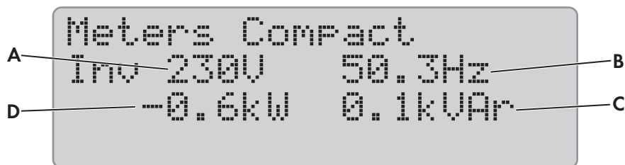
Abbildung 16: Übersicht des Menüs Meters Compact für die AC-Messwerte des Wechselrichters Sunny Island
