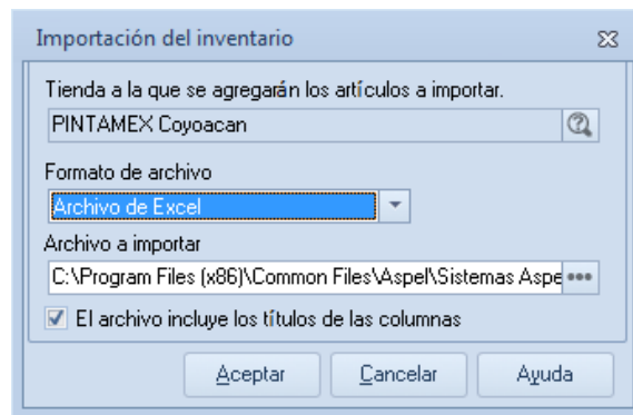
Figura 4. Tienda, formato y ruta del archivo a importar.
