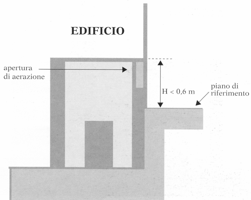
Tavola 2c - Locale interrato
