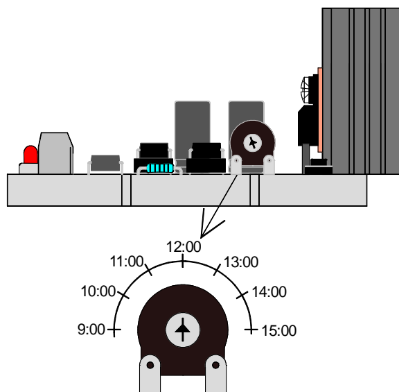
Abbildung 1: Potentiometer P1 „Steuertakt“.
