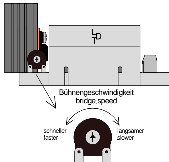
Abbildung 2: Potentiometer P2 „Bühnengeschwindigkeit (Speed)“.
