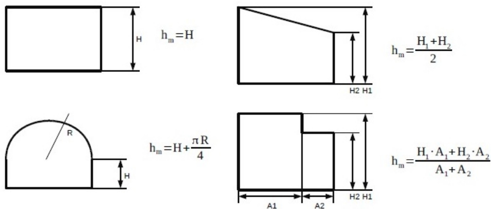
Illustrazione G.1-2: Esempi di determinazione dell'altezza media
