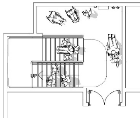
Illustrazione S.4-5: Esempio di spazio calmo (area of rescue assistance) secondo ISO 21452
