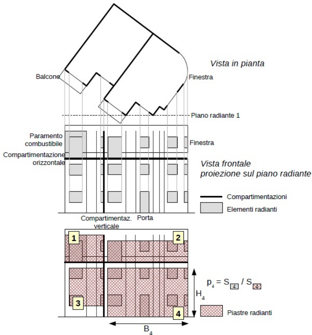
Illustrazione S.3-3: Determinazione delle piastranti, vista in pianta e frontale
