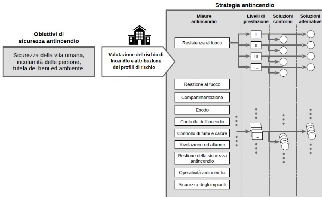
Illustrazione G.2-1: Schematizzazione della metodologia generale
