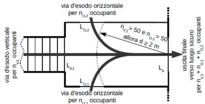
Illustrazione S.4-4: Flussi d'esodo convergenti (merging flows) verso uscita finale, in pianta
