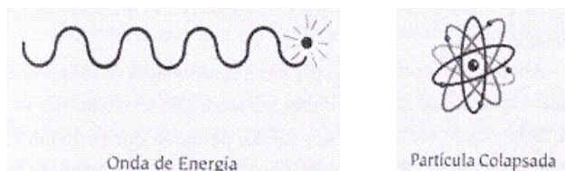
Fig 14: La Onda de Energía Colapsando en una Partícula
