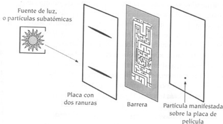
Fig. 16: El Experimento de la Doble Ranura
