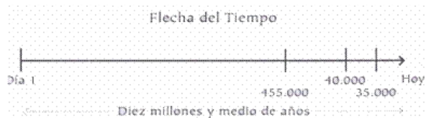
Fig 21: La Flecha del Tiempo
