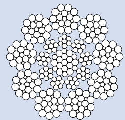
Fig. 23: DRAKO 300T, 9x25F + IWRC
