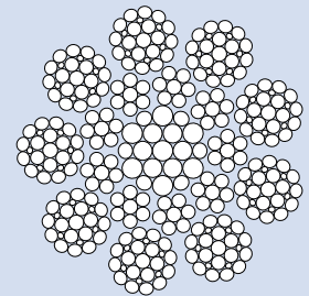
DRAKO 300TP
