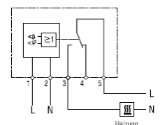
Anschlussdiagramm
